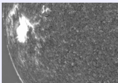
Цунами на Солнце
