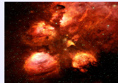
Туманность Кошачья Лапа
