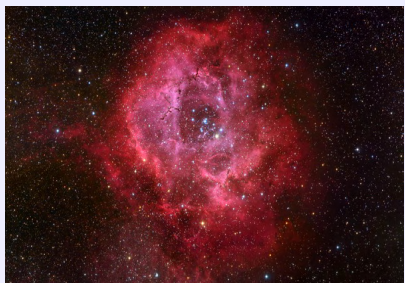
Туманность Розетка. Роза
