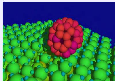
Фуллерины
