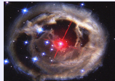
Световое эхо от V838
