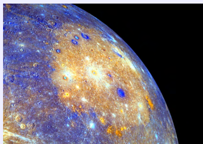
Меркурий. Кратер Калорис
