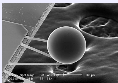
Эффект Казимира
