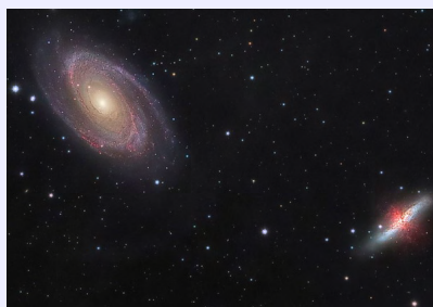
Галактические войны
