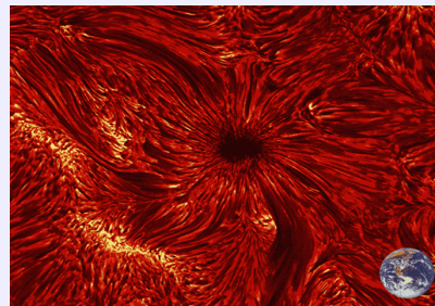
Превращение солнечного пятна
