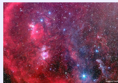
Пояс Ориона
