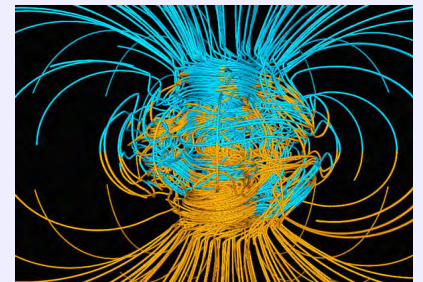
Магнитное поле Земли
