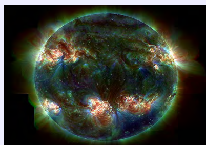
Темное палящее Солнце
