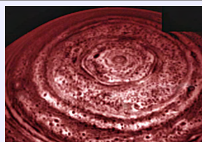
Облака на Сатурне
