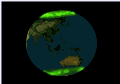
Полярные сияния Земли
