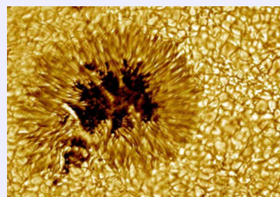
Солнечное пятно
