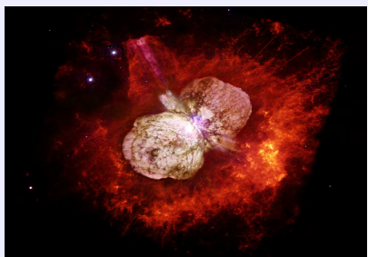
Звезда Киля
