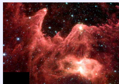
Горы созидания Кассиопеи
