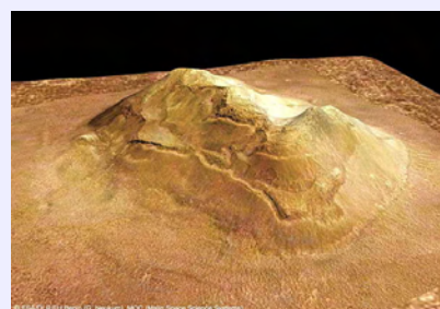
Снимок Лица на Марсе
