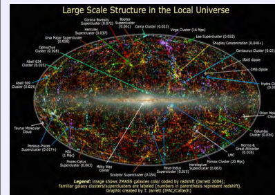
Ближняя Вселенная
